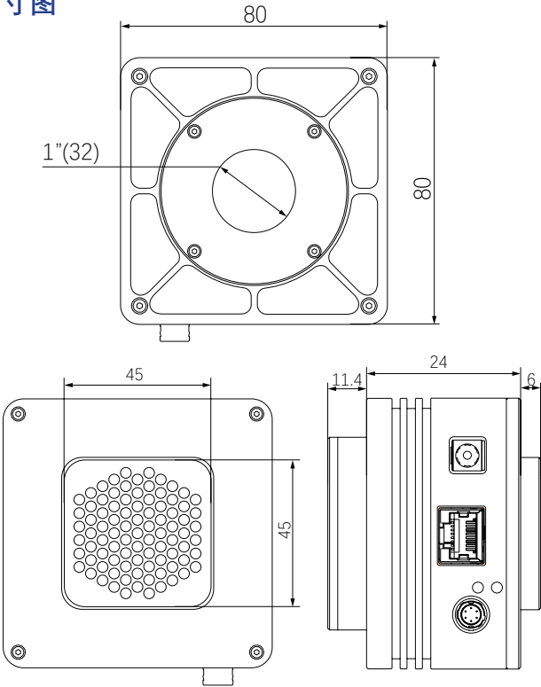
尺寸图
