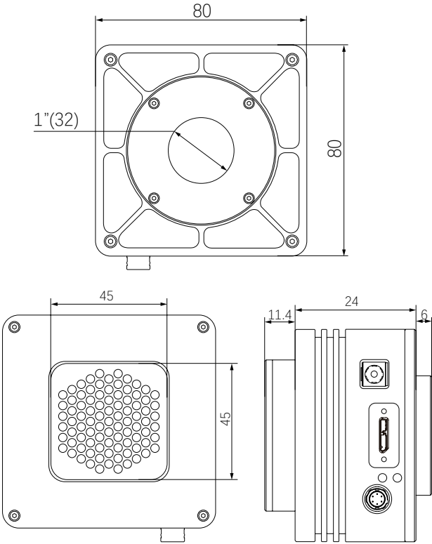
尺寸图
