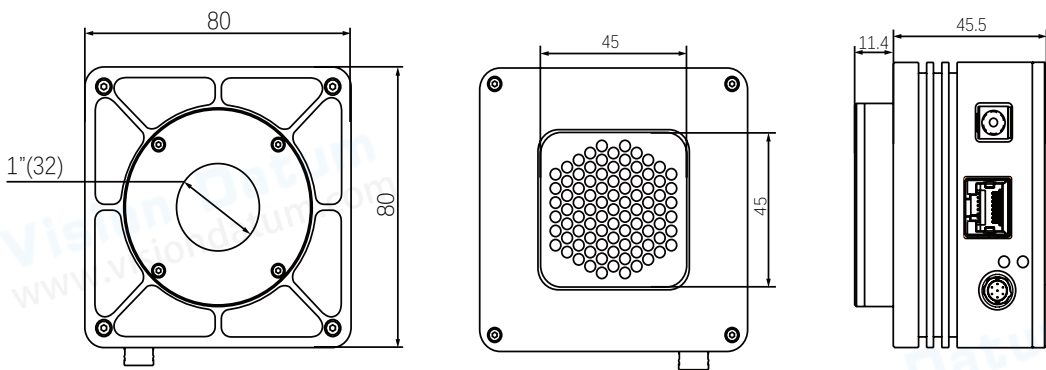
Dimensions B
