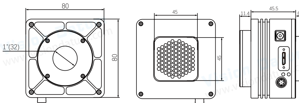
尺寸图 A
