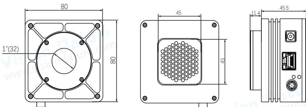
尺寸图 B
