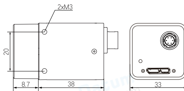
尺寸图 D
