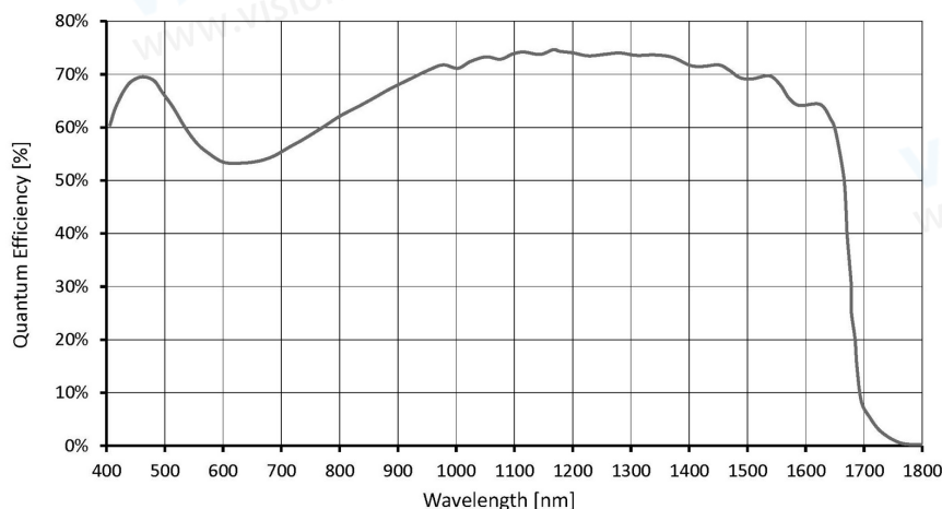
IMX990 绝对量子效率
