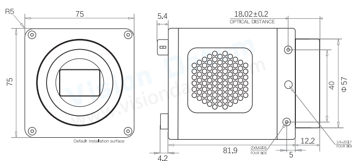
尺寸图 C
