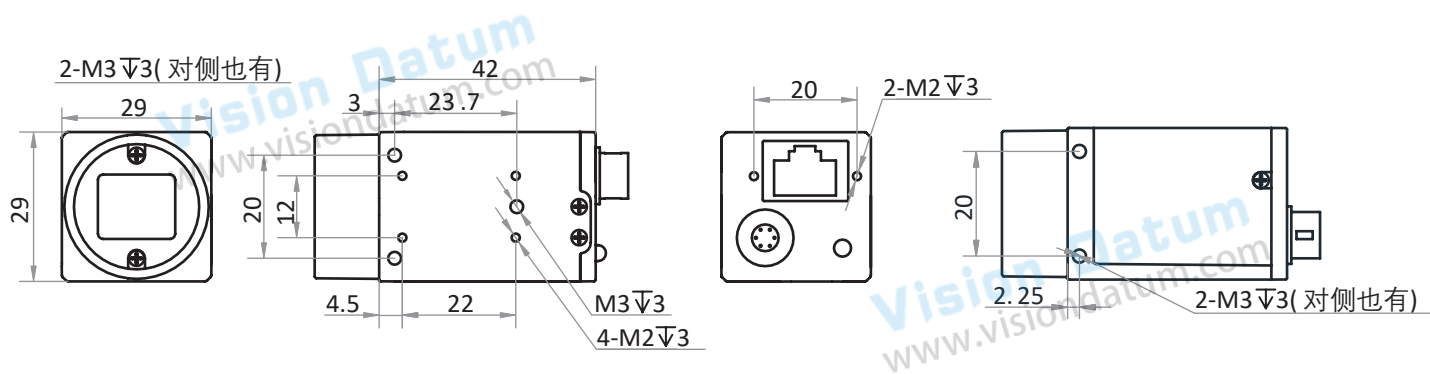
图 1-2: 29 * 29 * 42 mm 外壳的 C 口 GigE SWIR 相机的机械尺寸（以 mm 为单位），安装采用 M2、M3 规格螺丝。
