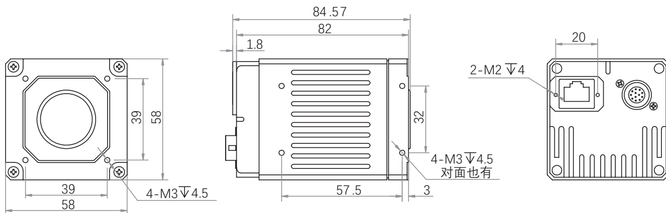
图 1-1: 58 * 58 * 82 mm 外壳的 C 口 GigE SWIR 相机的机械尺寸（以 mm 为单位），安装采用 M2、M3 规格螺丝。
