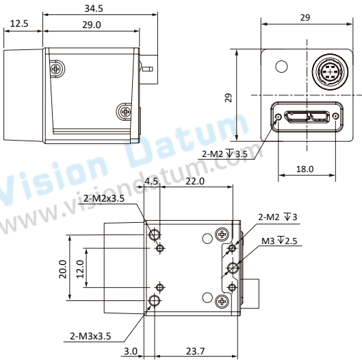
尺寸图
