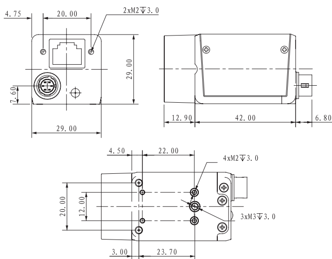
尺寸图
