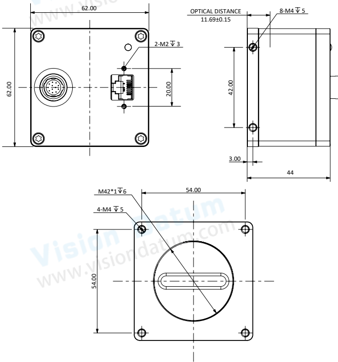
尺寸图
