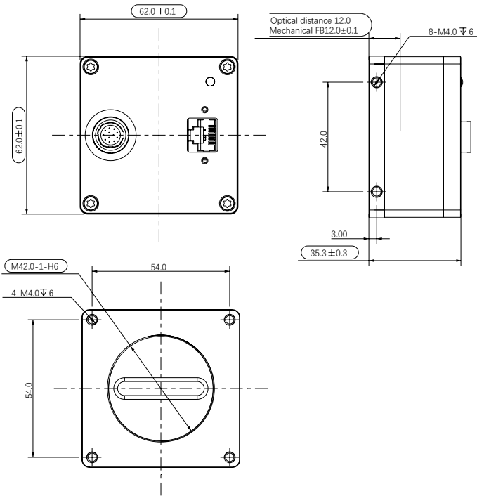
尺寸图
