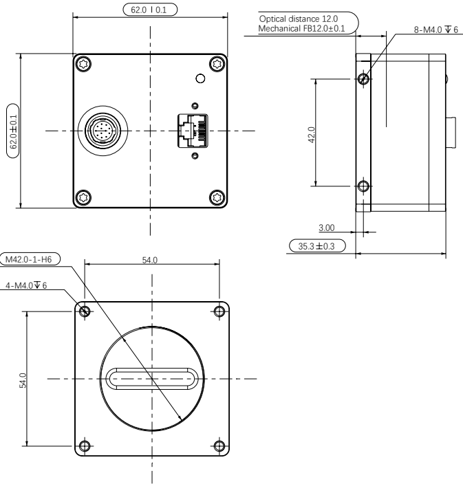
尺寸图
