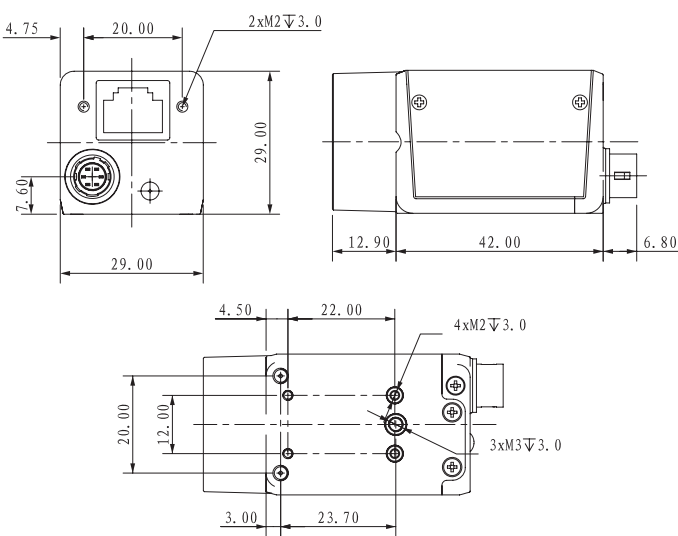
尺寸图
