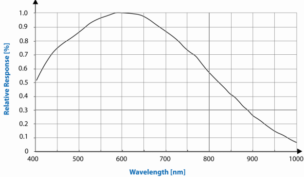
光谱响应
