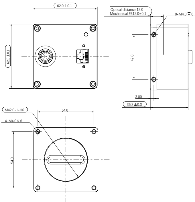
尺寸图
