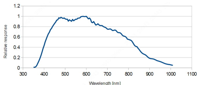
光谱响应
