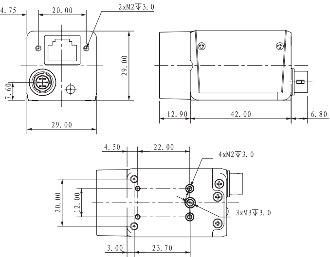
尺寸图
