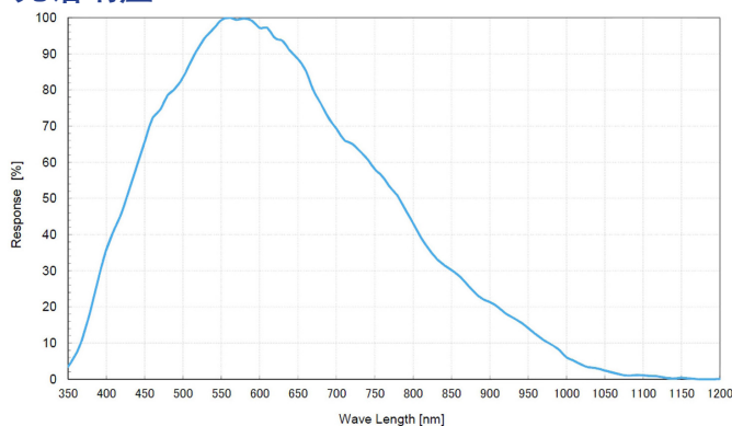
光谱响应
