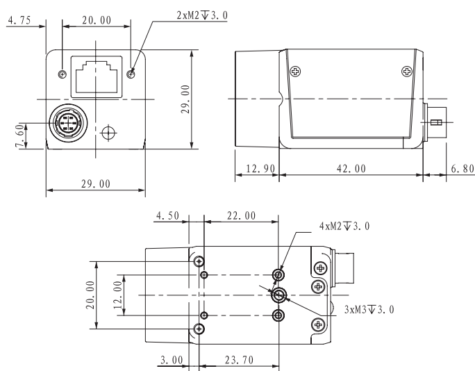
尺寸图
