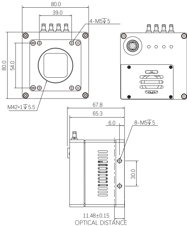
尺寸图
