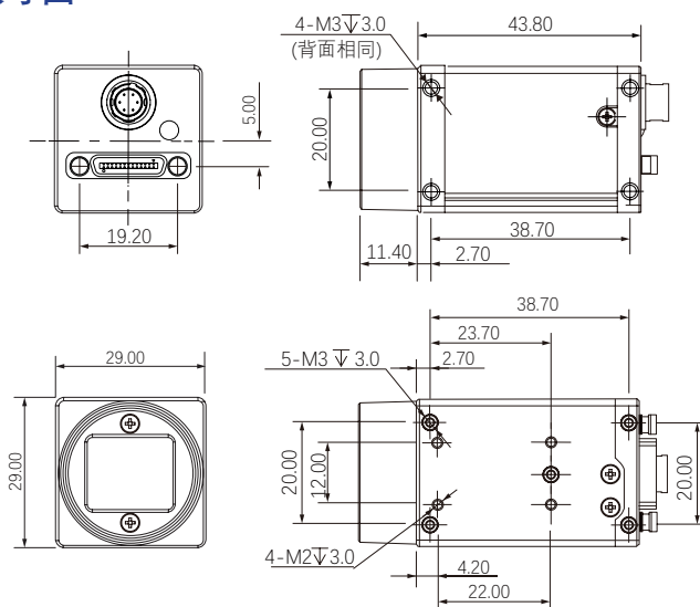
尺寸图
