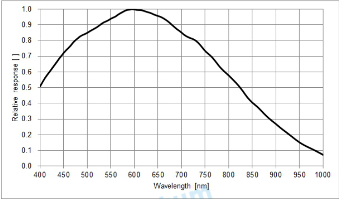
光谱响应
