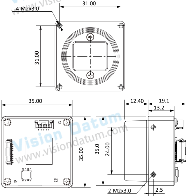
尺寸图
