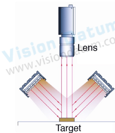
光源结构图
