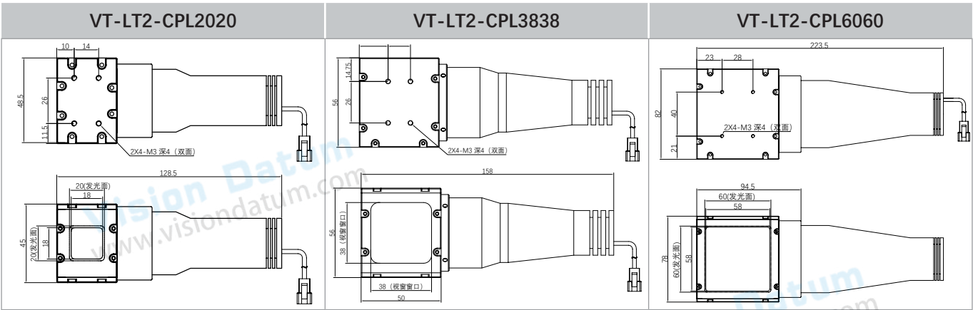
尺寸图 (mm)
