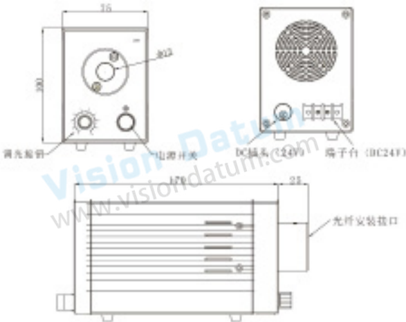
尺寸图 (mm)
