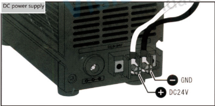
将背面的端子块插入 24V DC 电源
