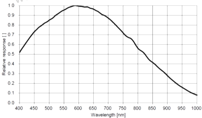
光谱响应
