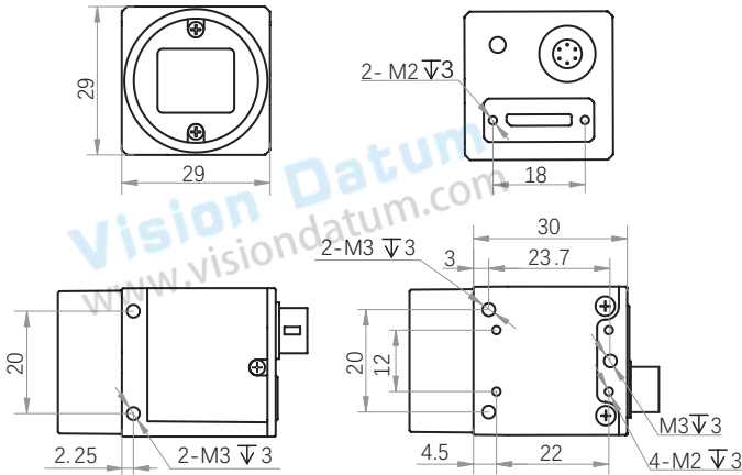
尺寸图
