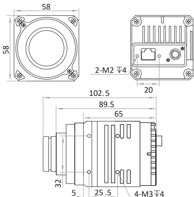
尺寸图
