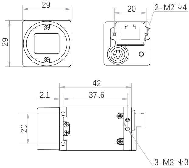
尺寸图
