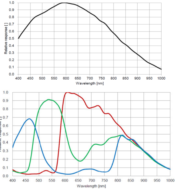
光谱响应
