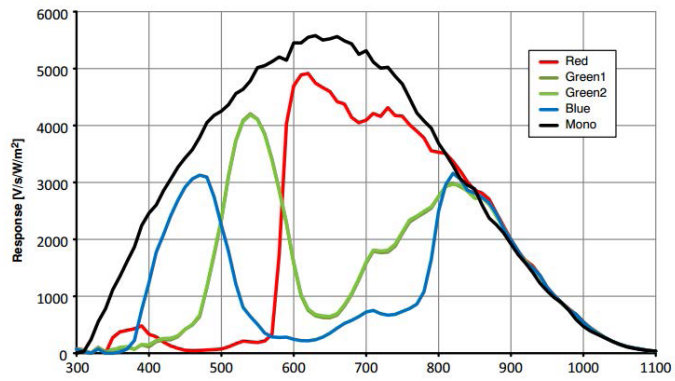
光谱响应
