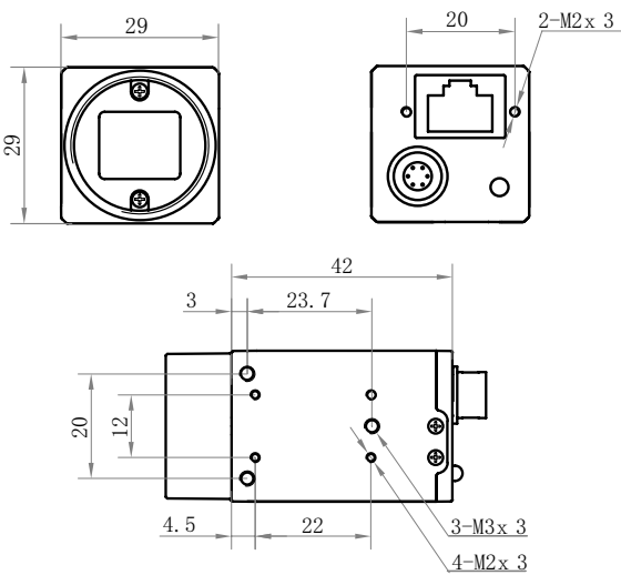
尺寸图
