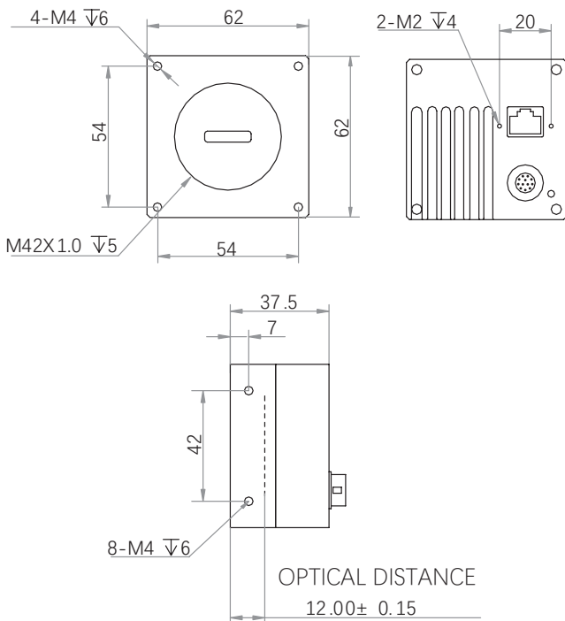
尺寸图
