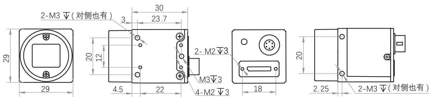
图 1-3: 29 mm×29 mm×30 mm，四面可固定的 USB3.0 相机的机械尺寸（以 mm 为单位）。
