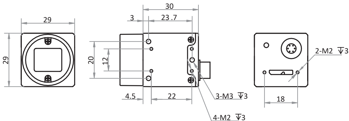
图 1-1: 29 mm×29 mm×30 mm，USB 接口在下的 USB3.0 相机的机械尺寸（以 mm 为单位）。
