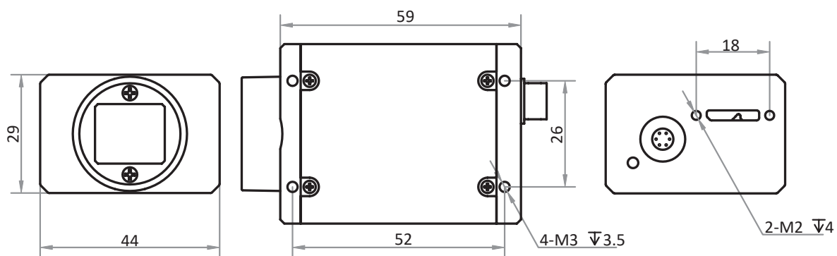
图 1-5: 29 mm×44 mm×59 mm, USB3.0 相机的机械尺寸 (以 mm 为单位)。
