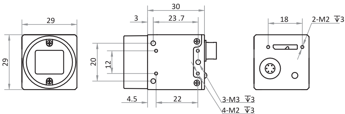
图 1-2: 29 mm×29 mm×30 mm，USB 接口在上的 USB3.0 相机的机械尺寸（以 mm 为单位）。
