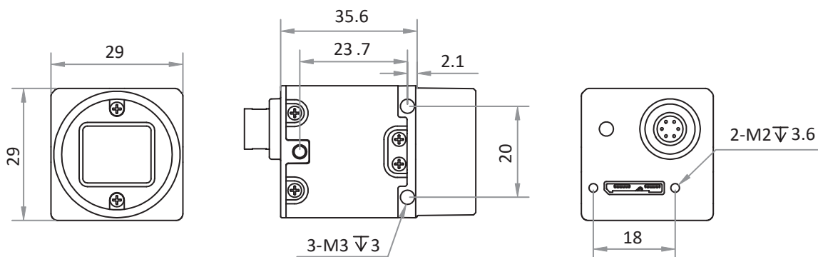
图 1-4: 29 mm×29 mm×30 mm，USB 接口在下的 USB3.0 相机的机械尺寸（以 mm 为单位）。
